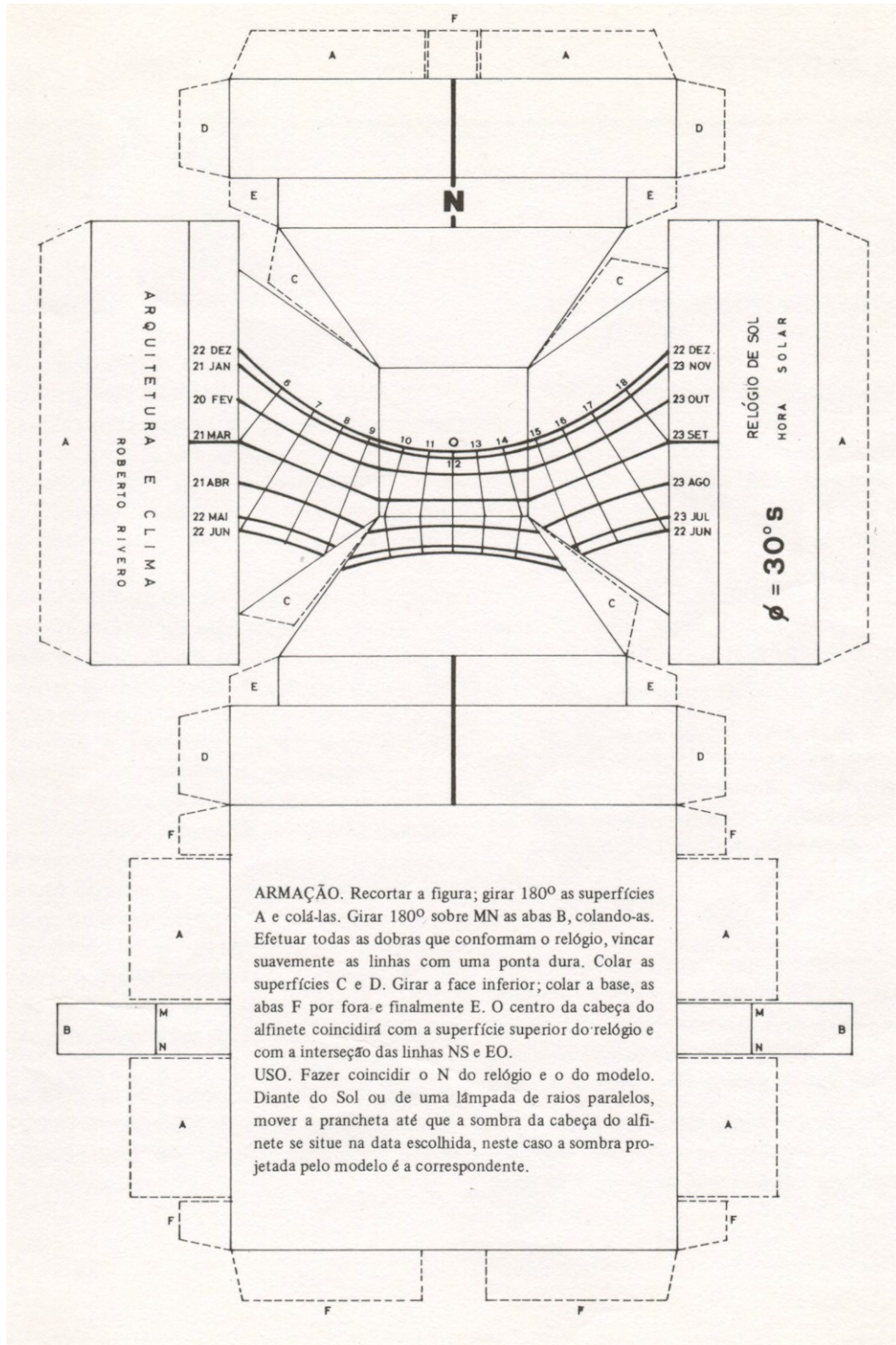
RELÓGIO DE SOL PARA A LATITUDE 30° S Fonte: Rivero
