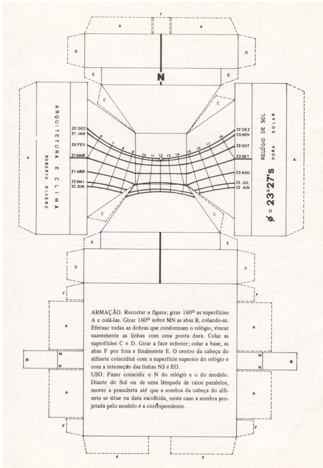
RELÓGIO DE SOL PARA A LATITUDE 23^{\circ}27' S
